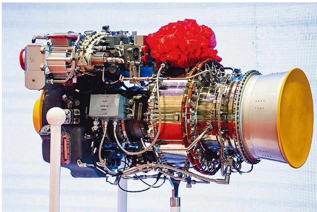
航空发动机及燃气轮机是“十四五”规划 102 项重大工程项目之一。AES100 发动机是我国第一型严格按照国际通行适航标准自主创新研制的 1000 千瓦级民用涡轴发动机。2025 年 6 月 5 日在湖南省株洲市举办的 AES100 发动机研制工作总结会宣布，AES100 发动机获颁生产许可证。图为当日拍摄的 AES100 发动机。新华社记者 陈思汗/摄
